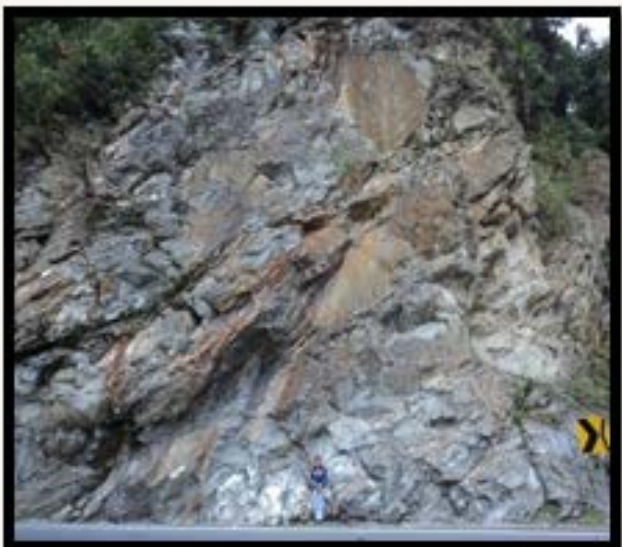
Fotografía 1: Augens de deformación en esquistos micáceos, ubicada aproximadamente a 200 m de la estación de bombeo de Baeza (UTM: 838197; 9952130; 2138 m.s.n.m.) Tomada por: Andrea García, (2014).
