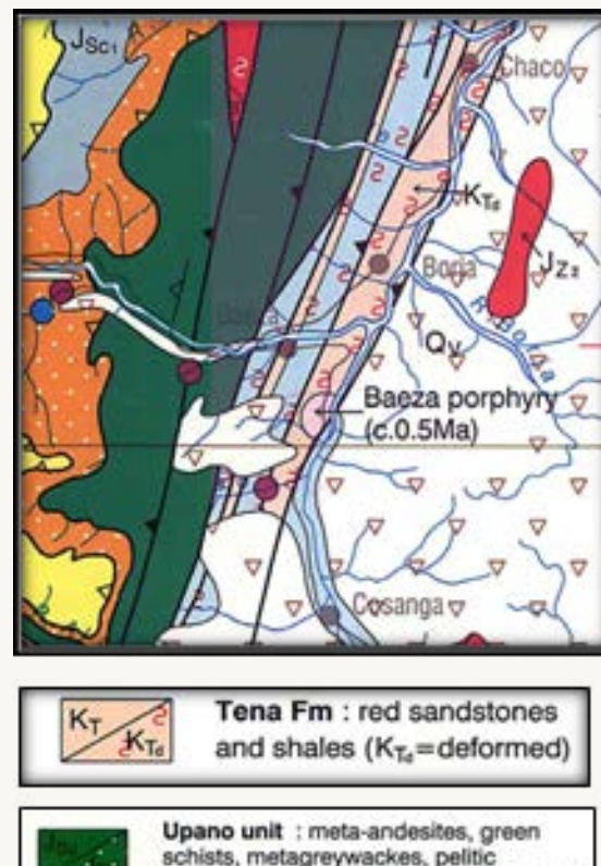
Figura 2. Sección del mapa geológico de la Cordillera Real (Norte). Tomado de Geological and Metal Occurrence Maps of the Northern Cordillera Real Metamorphic Belt. (1994).
