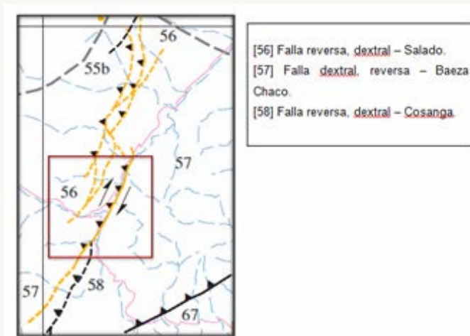
Figura 3. Fallas activas que se encuentran en la zona de estudio. Tomado de U.S.G.S., E.P.N., (2003). Mapa de Fallas y Pliegues Cuaternarias de Ecuador y Regiones Oceánicas Adyacentes.
