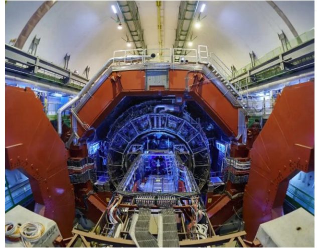
Figura 3. ALICE es uno de los principales detectores del Gran Colisionador de Hadrones (LHC) del CERN. Con 26 m de diámetro y 16 m de largo, fue diseñado para estudiar colisiones de iones pesados, como el plomo. Está ubicado a 56 metros de profundidad en una gran caverna subterránea, cerca del pueblo de Saint-Genis-Pouilly, en Francia (CERN,2025).
