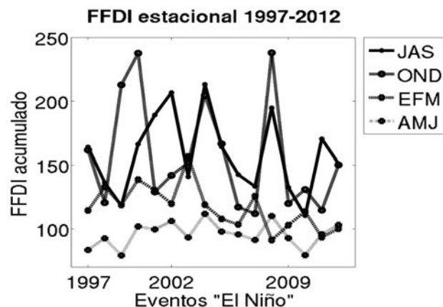
Figura 4: Serie de tiempo del Índice de Peligro de Incendios Forestales FFDI estacional para los períodos julio-agosto-septiembre (JAS), octubre-noviembre-diciembre (OND), enero-febrero-marzo (EFM), Abril-Mayo-Junio (AMJ) en la región andina de Ecuador para el período 1997-2012. Las temporadas JAS y OND son las que evidencian un riesgo más alto de ocurrencia de incendios forestales.
