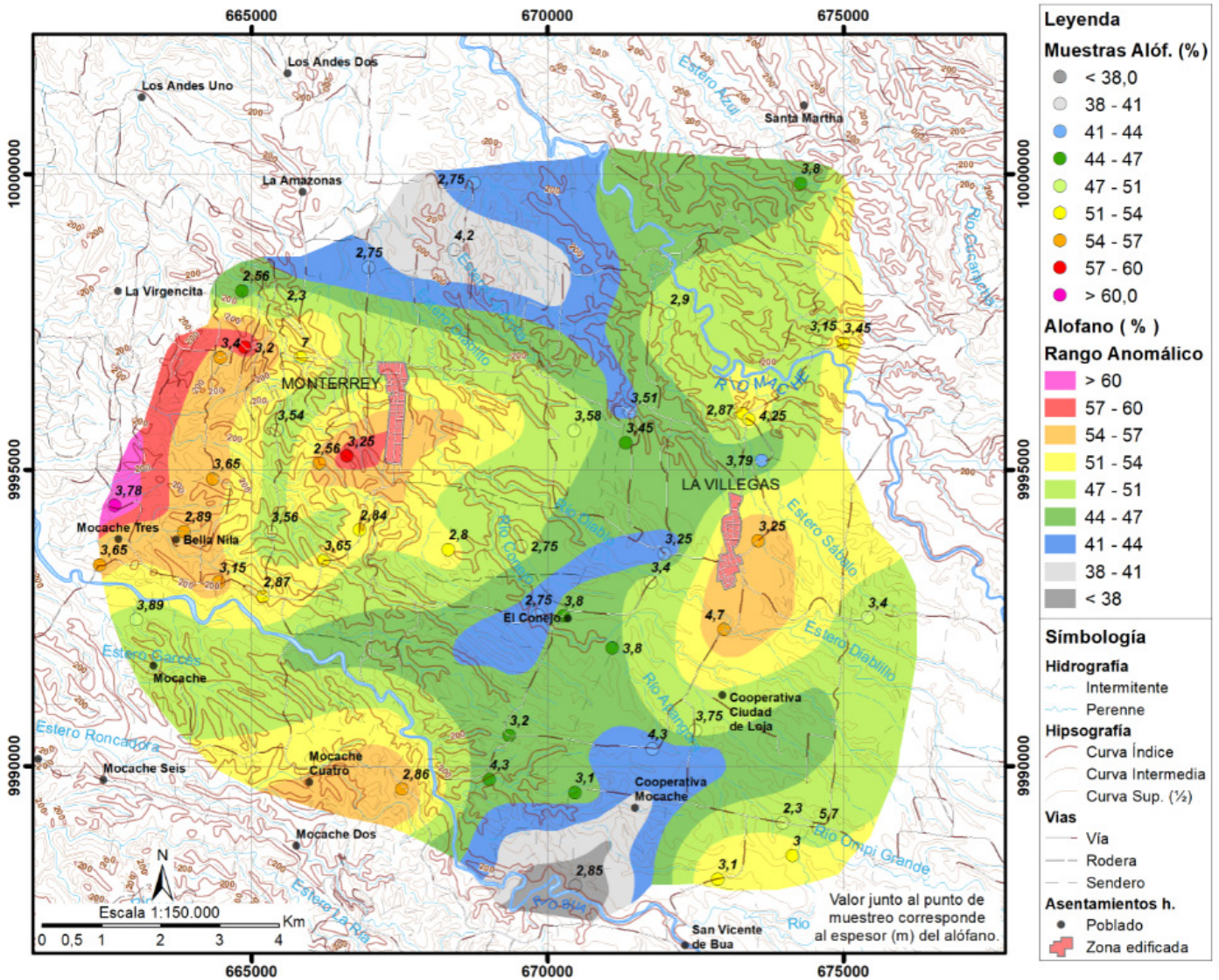
Figura 4. Mapa de zonas anomálicas de alófono. Monterrey. Provincia de Santo Domingo de los Tsáchilas.
