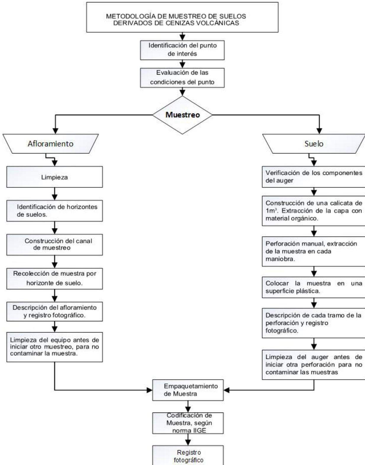
Figura 3. Metodología de muestreo de suelos derivados de cenizas volcánicas, basado en la norma ANSI. / Fuente: IIGE, 2020
