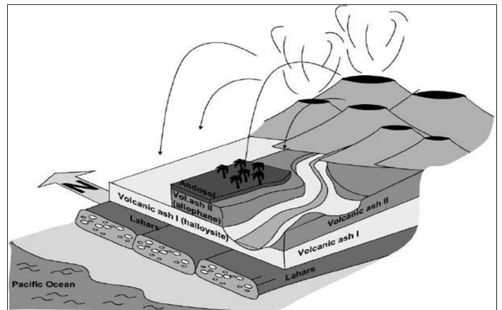
Figura 2. Sección idealizada del ambiente geológico en el que se desarrolla la capa rica en alófono.
