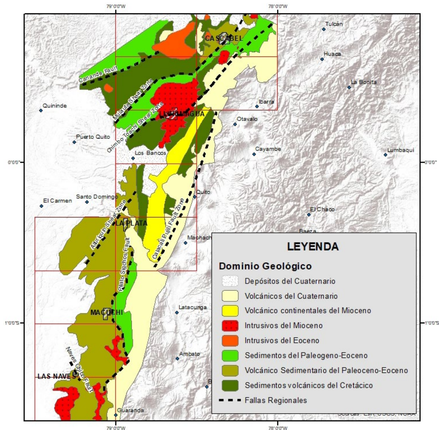
FIGURA 3 Mapas de dominios geológicos y fallas
