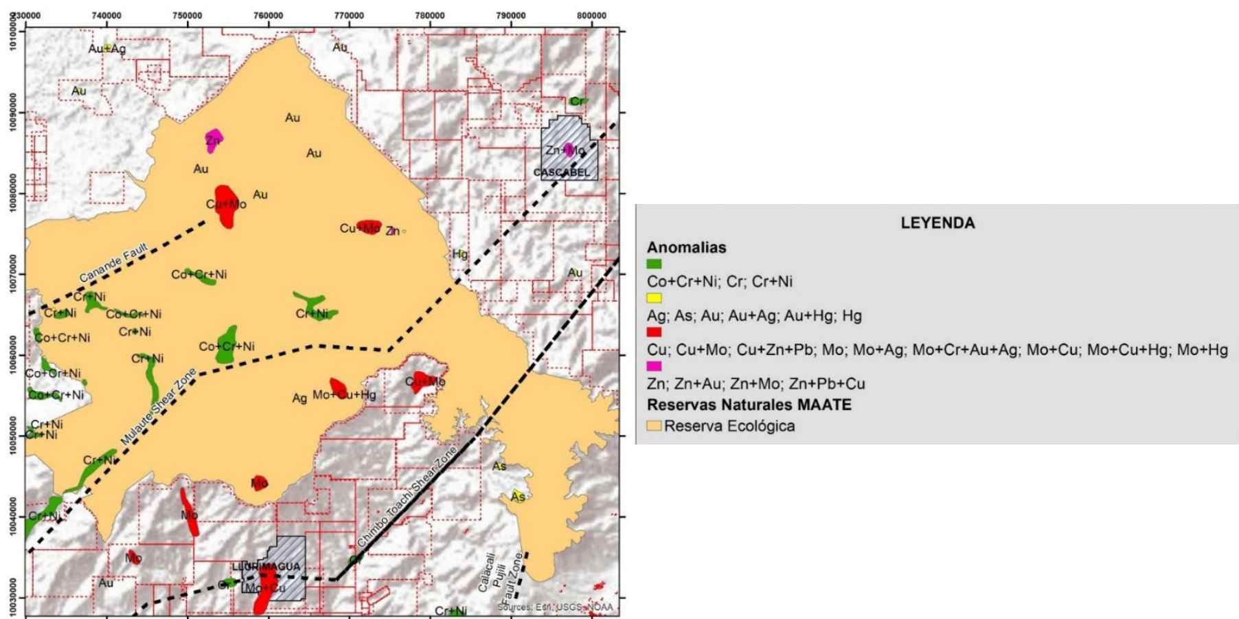
FIGURA 5 Mapa consolidado de anomalías, reservas y concesiones
