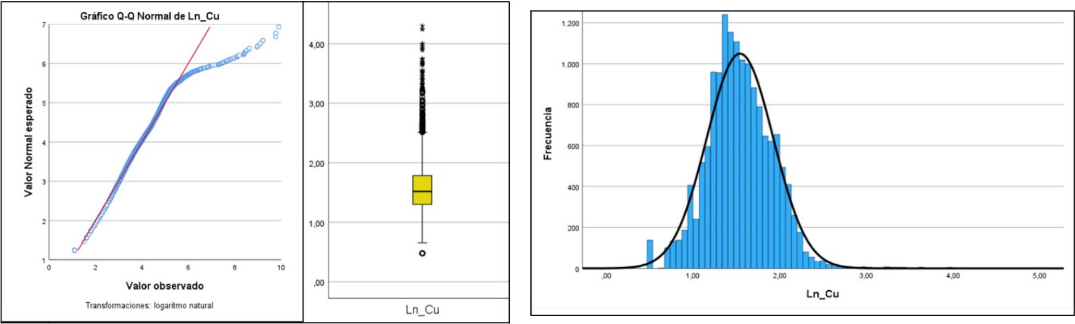
FIGURA 1 Gráficos para la estadística descriptiva del cobre
