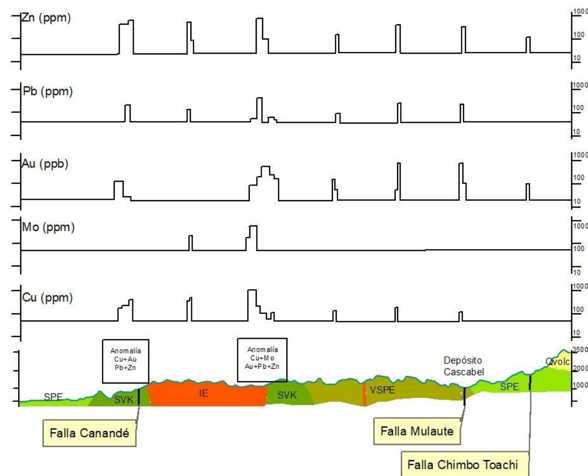
FIGURA 8 Corte 2 de la Cordillera Occidental
