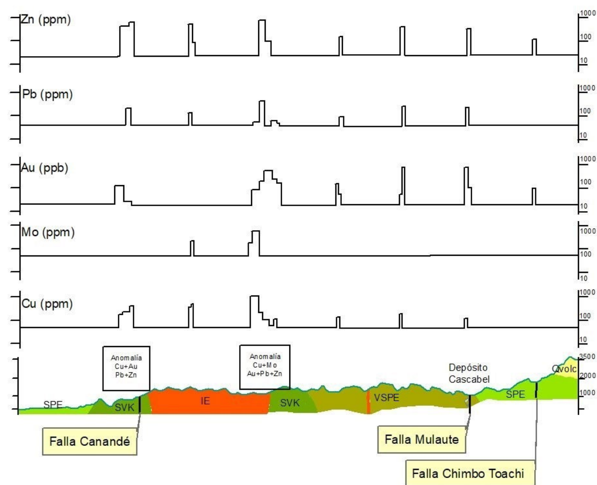
FIGURA 7 Corte 1 de la Cordillera Occidental
