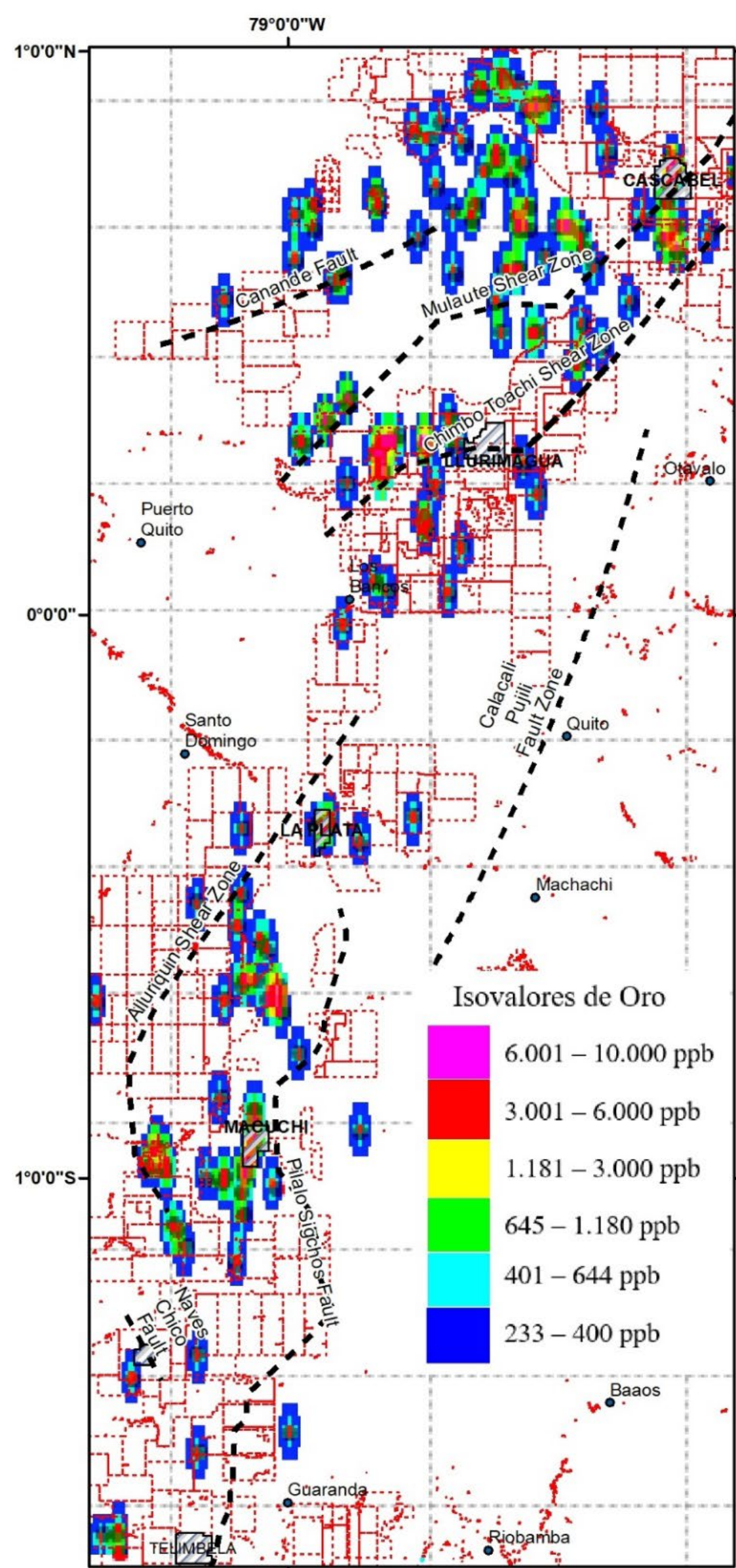
FIGURA 2 Mapa de anomalías de Au en ppb
