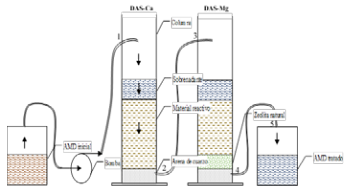
Figura 2. Diseño del sistema de tratamiento pasivo.
